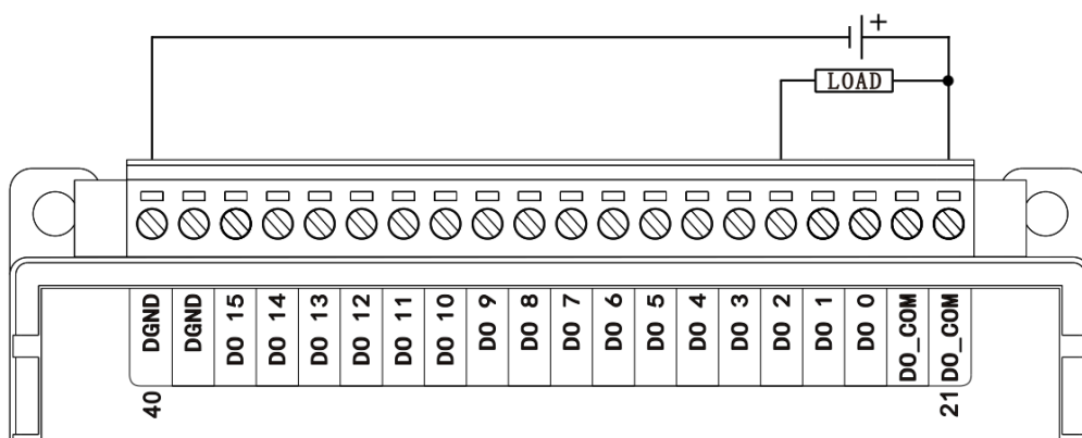
图 3-33 WTD650C 数字量输出接线方式
