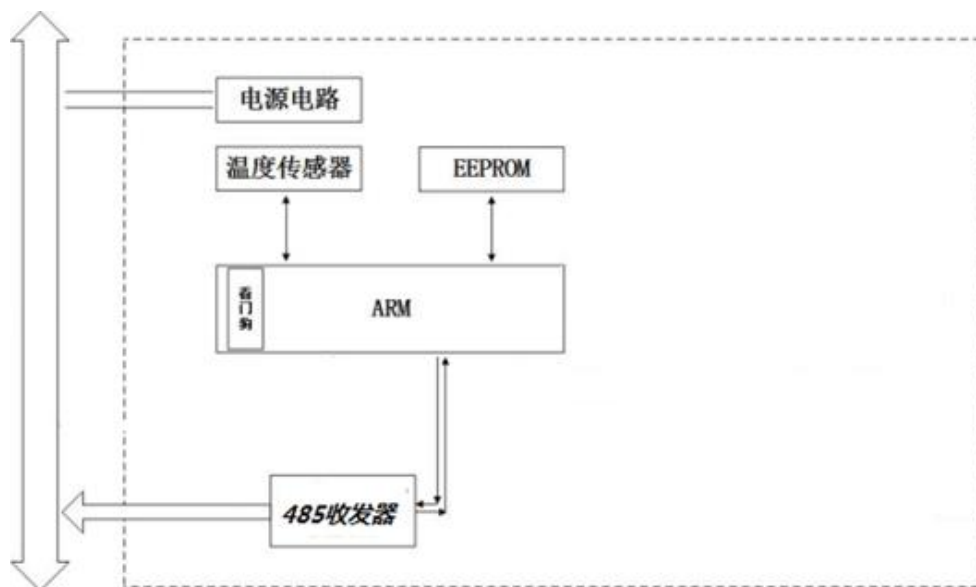
图 3-47 WTD634G 原理框图
