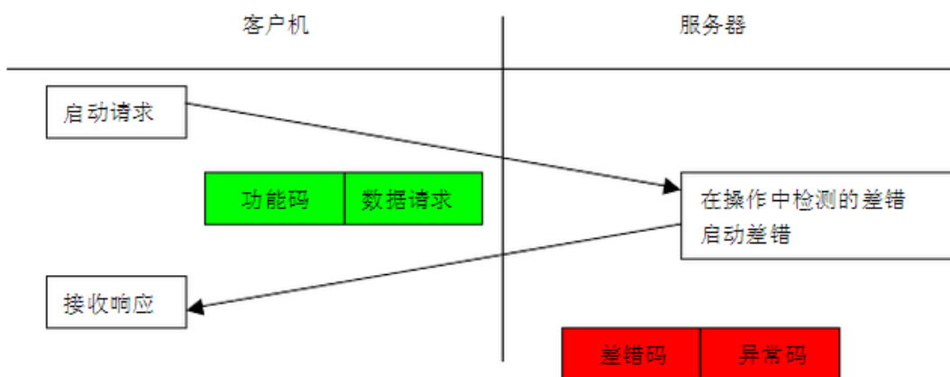
图 4-2 MODBUS 事务处理图(无差)
