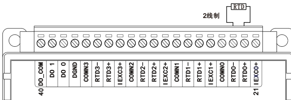
图 3-4 WTD614P 2 线 RTD 接线方式
