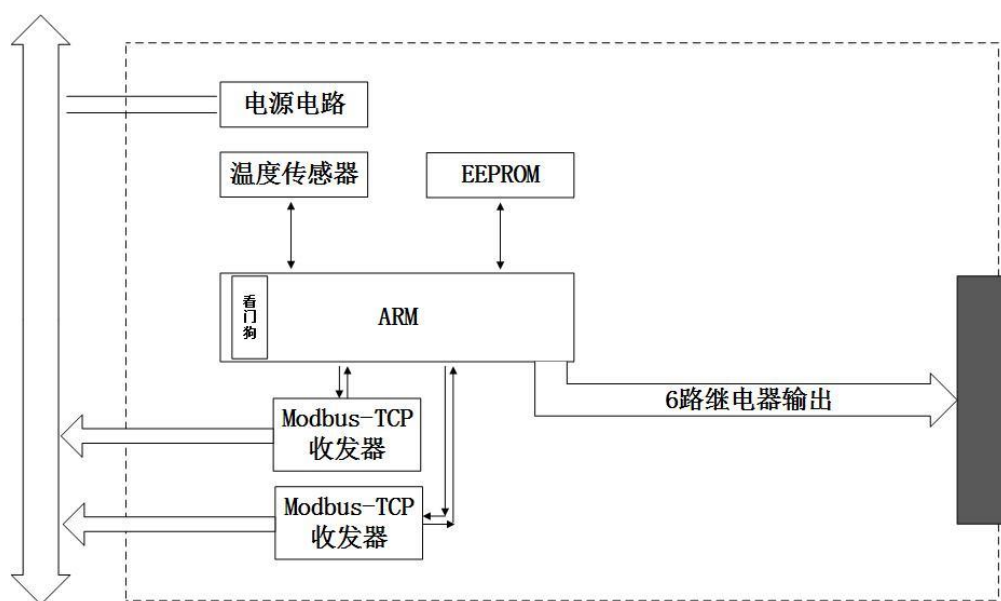
图3-35 WTD666C模块的原理框图
