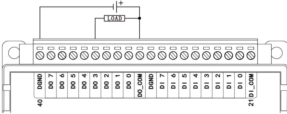
图 3-45 WTD678C 数字量输出接线方式
