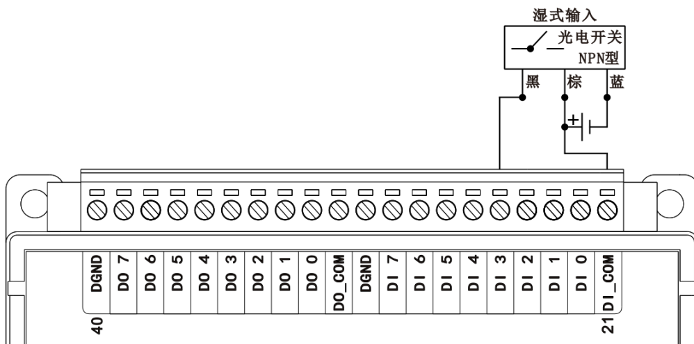
图 3-43 WTD678C NPN 型湿式输入接线方式
