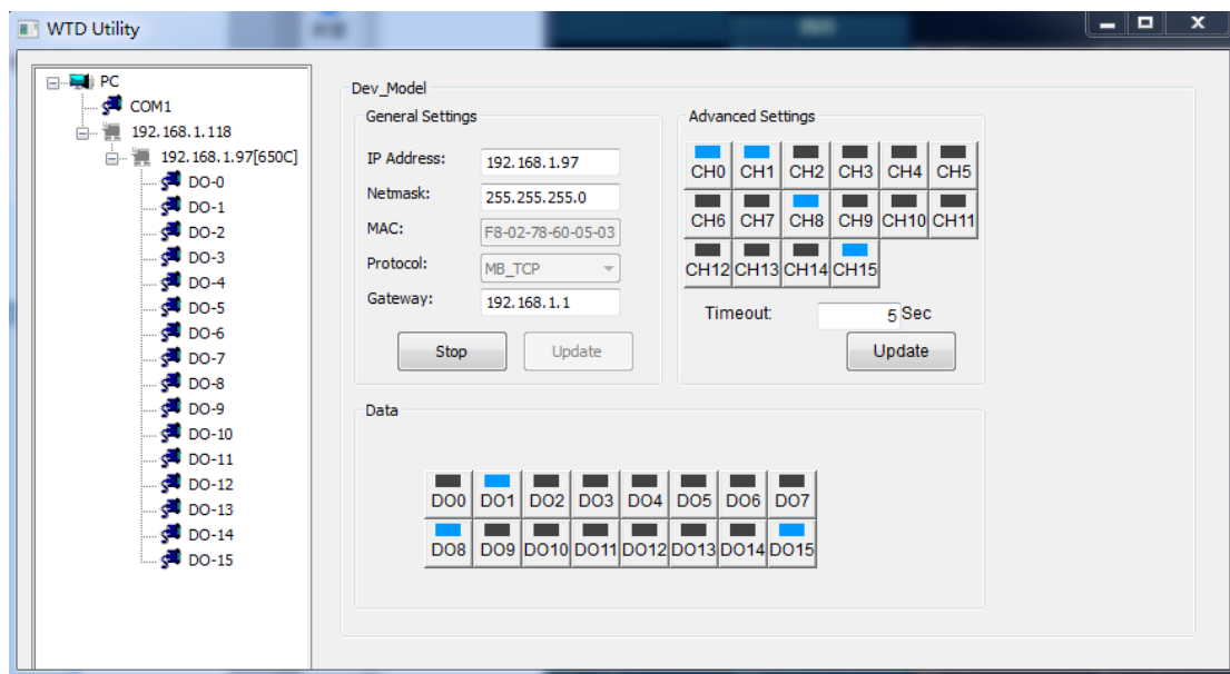
图 2-23 WTD650C 主界面
