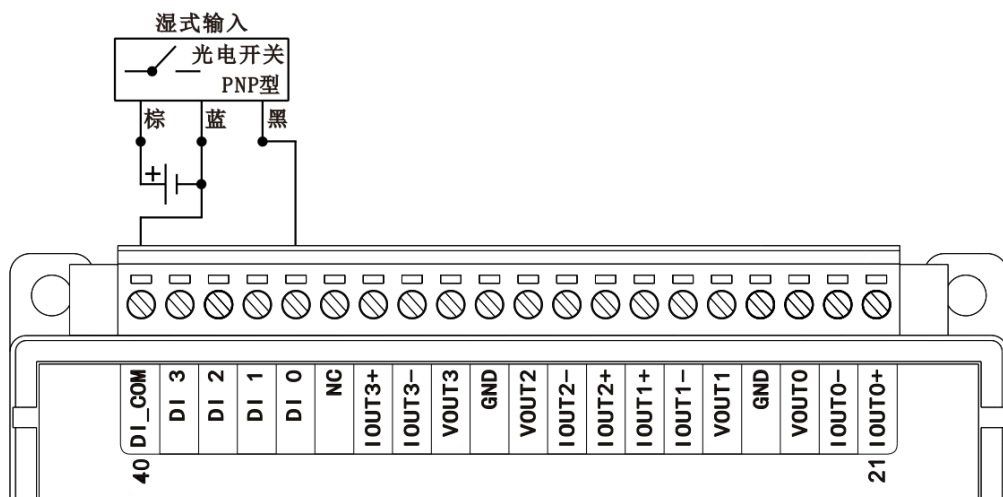
图 3-22 WTD624X PNP 型湿式输入接线方式
