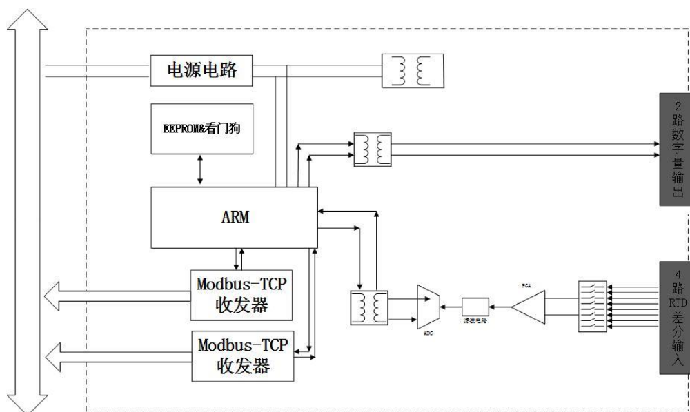
图 3-2 WTD614P 原理框图
