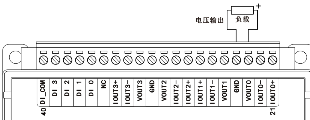
图 3-18 WTD624X 电压输出接线方式
