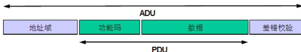
图 4-1 Modbus 协议帧
