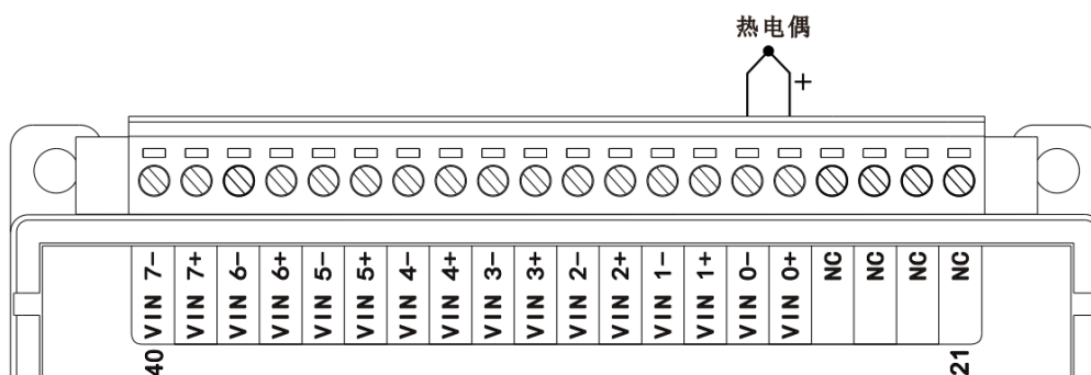
图 3-14 WTD618X 热电偶输入接线方式
