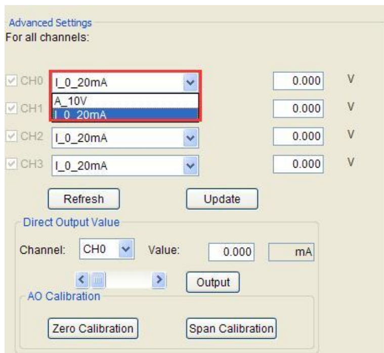
图 2-18 WTD624X 配置图
