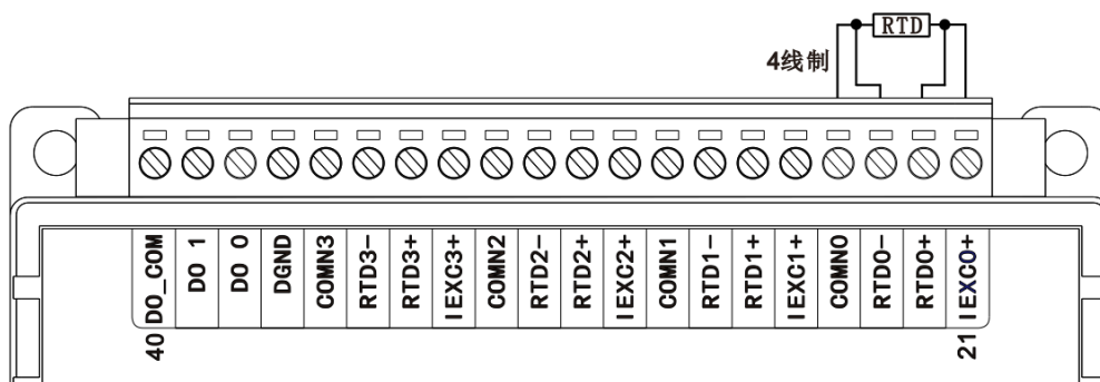
图 3-6 WTD614P 4 线 RTD 接线方式
