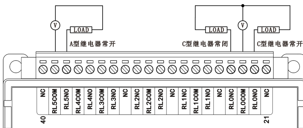
图 3-37 WTD666C 继电器输出接线方式
