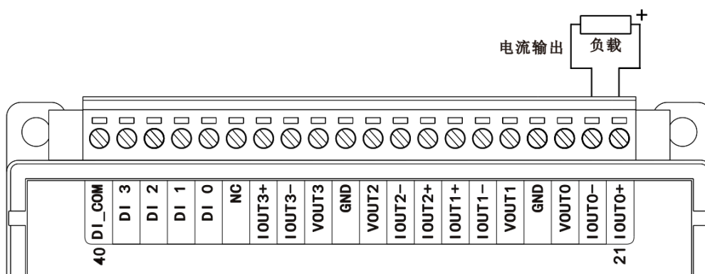
图 3-19 WTD624X 电流输出接线方式
