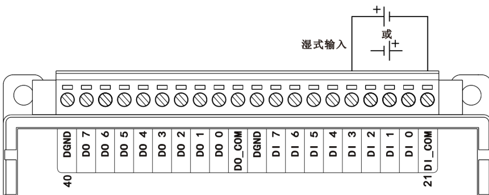
图 3-42 WTD678C 普通湿式输入接线方式
