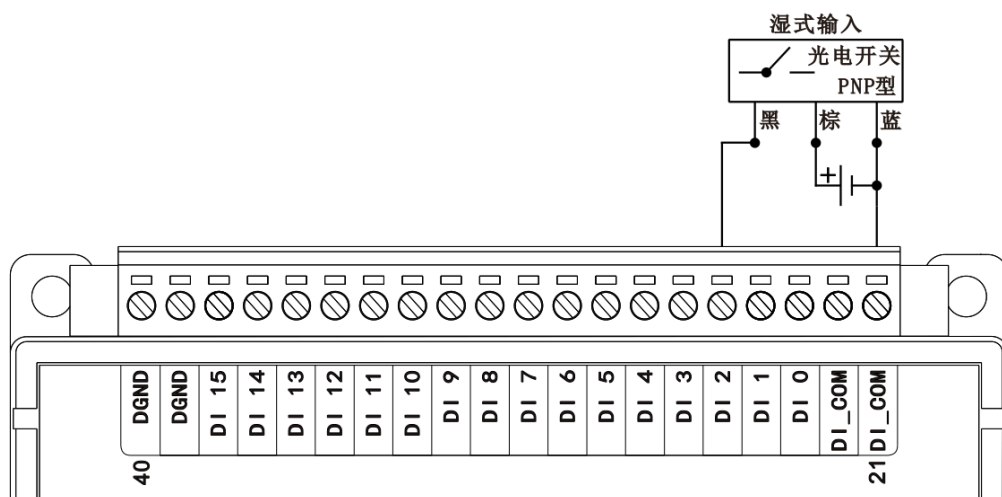
图 3-29 WTD640X PNP 型湿式输入接线方式
