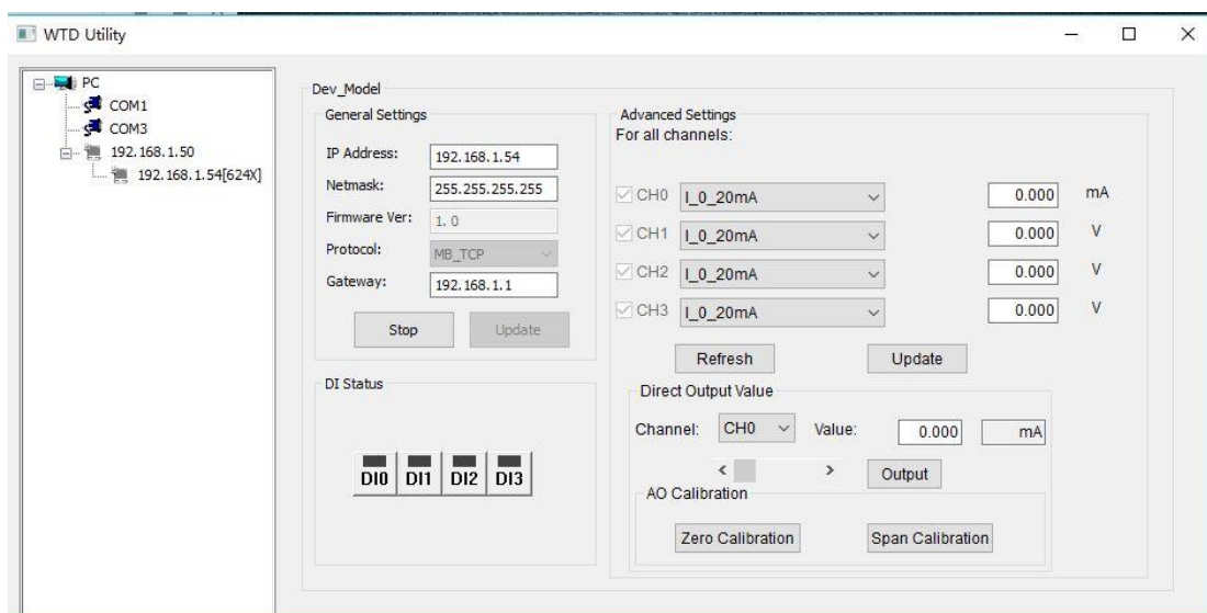
图 2-16 WTD624X 主界面
