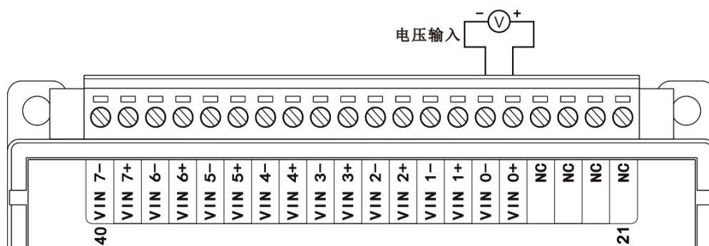
图 3-11 WTD618X 电压输入接线方式
