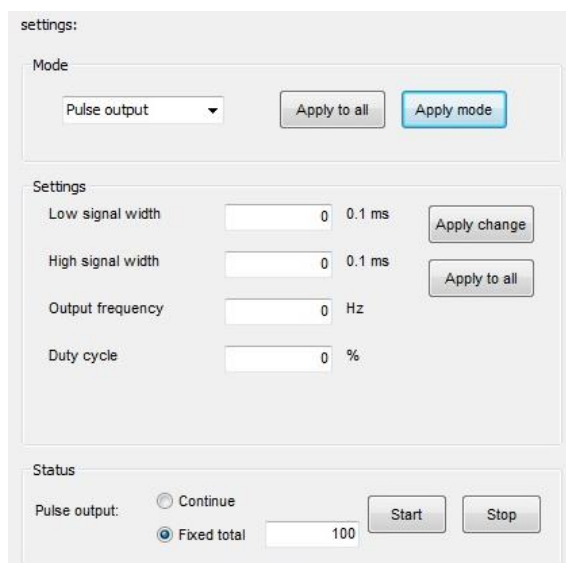
图 2-40 WTD678C 脉宽输出模式主界面
