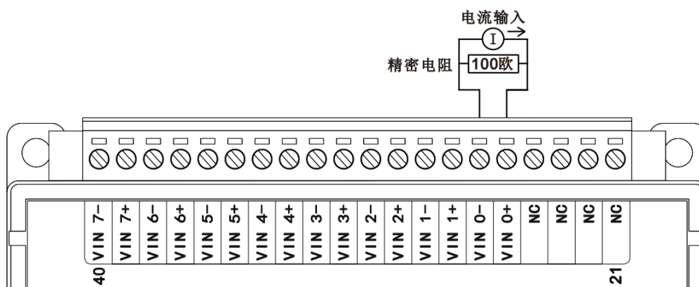
图 3-13 WTD618X 电流输入接线方式 2
