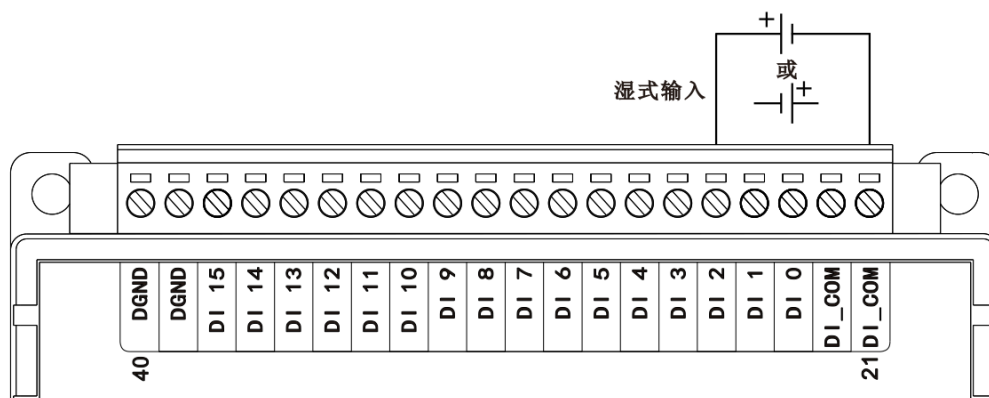
图 3-27 WTD640X 普通湿式输入接线方式
