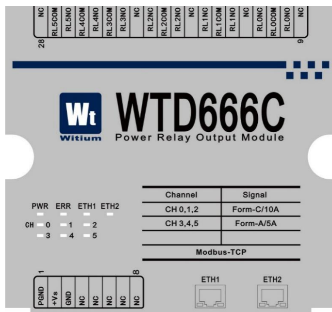
图 3-36 WTD666C 端子功能排列
