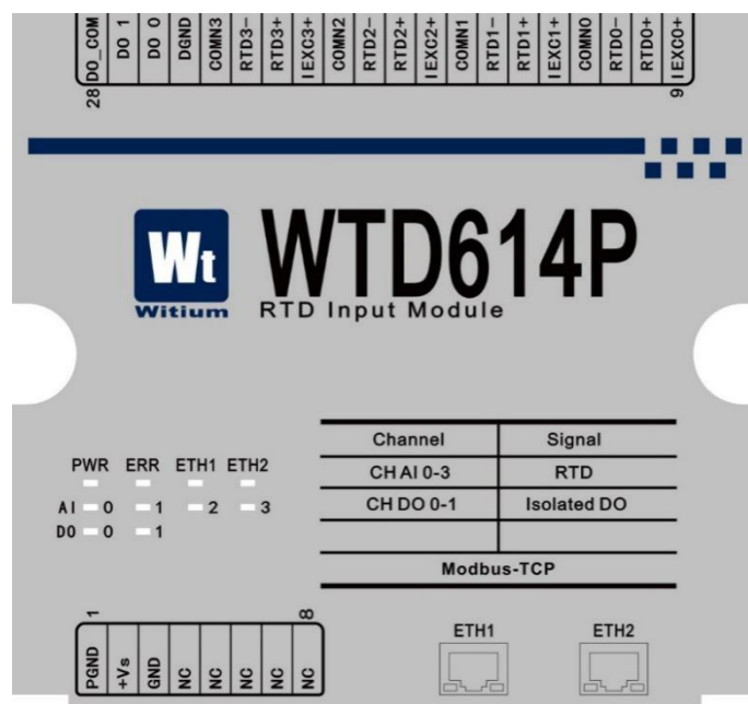
图 3-3 WTD614P 端子功能排列
