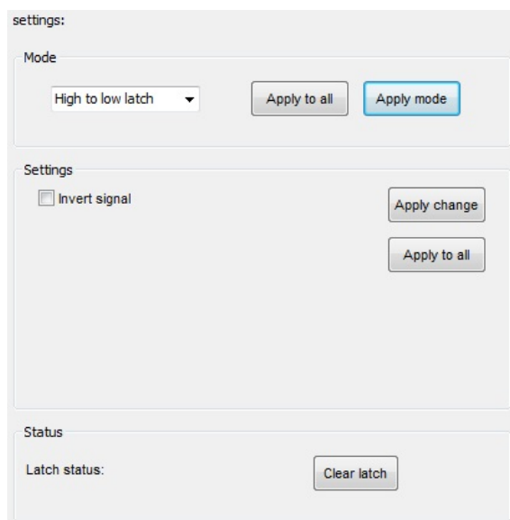
图 2-36 WTD678C 下降锁定模式主界面
