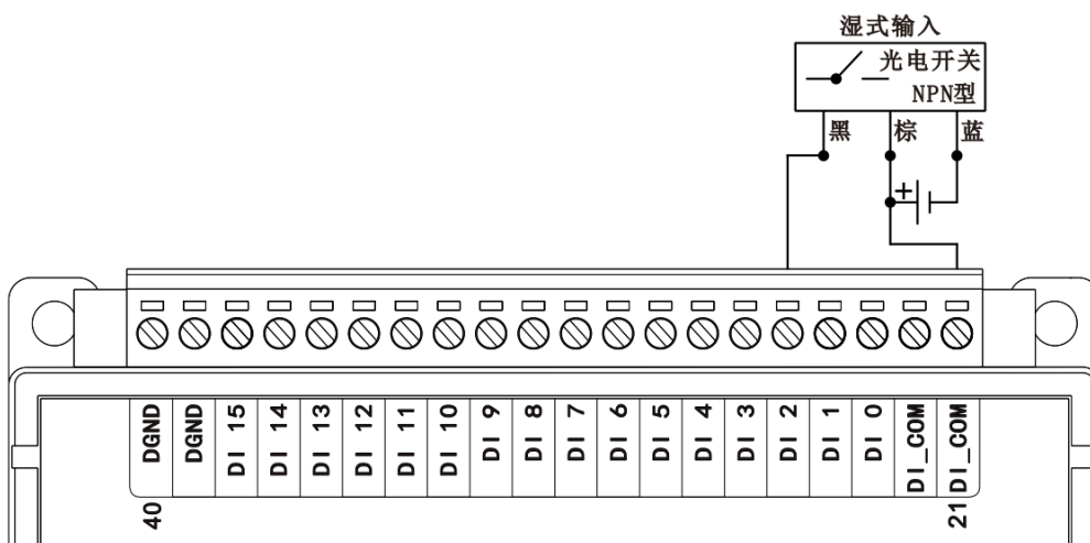
图 3-28 WTD640X NPN 型湿式输入接线方式
