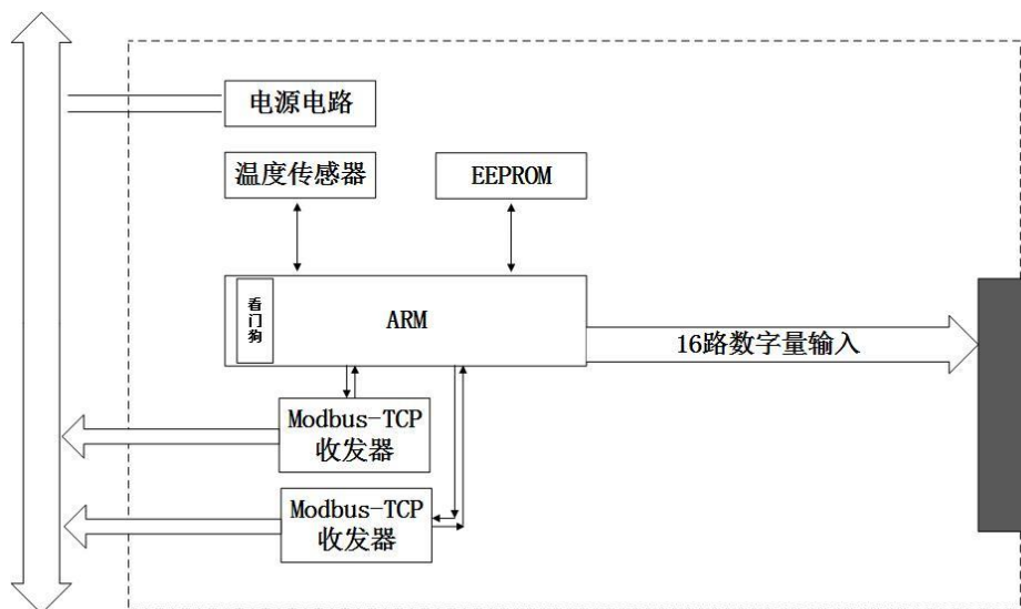
图 3-31 WTD650C 模块的原理框图
