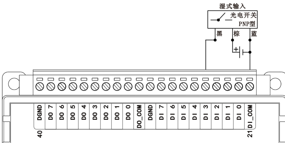
图 3-44 WTD678C PNP 型湿式输入接线方式
