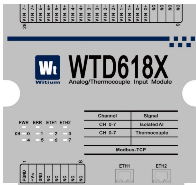
图 3-10 WTD618X 端子功能排列
