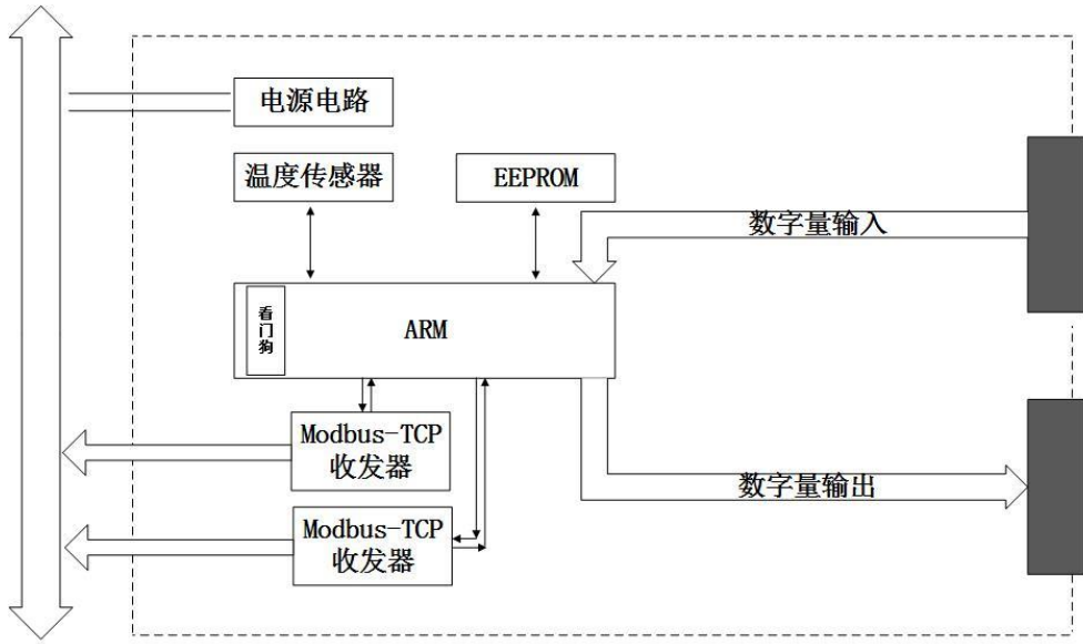
图 3-39 WTD678C 模块的原理框图
