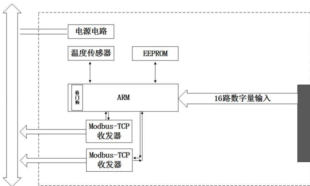
图 3-24 WTD640X 模块的原理框图
