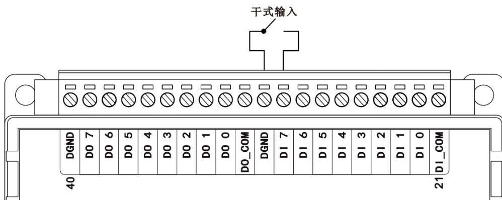
图 3-41 WTD678C 干式输入接线方式
