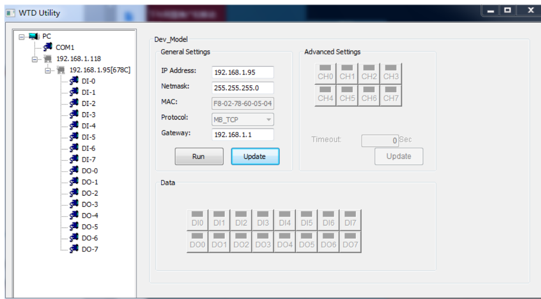
图 2-29 WTD678C 主界面
