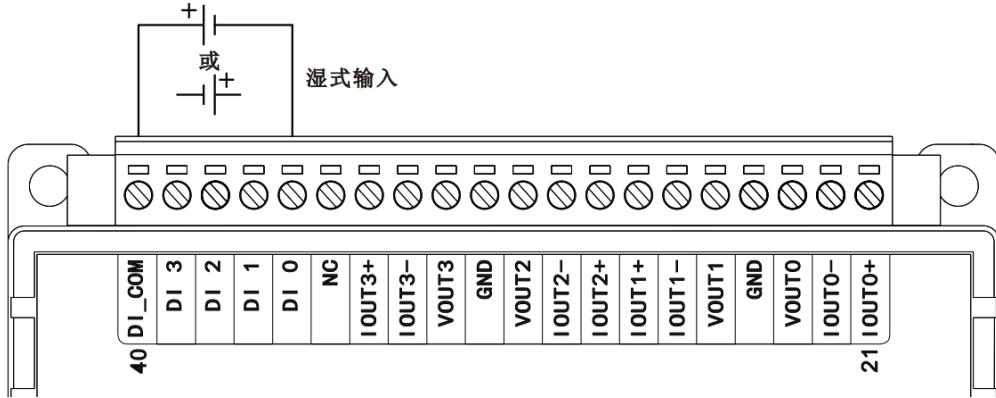
图 3-20 WTD624X 普通湿式输入接线方式
