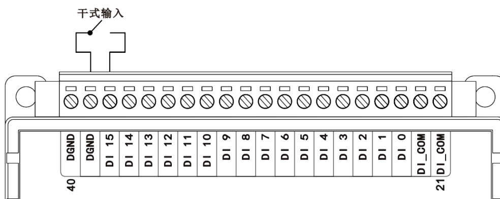
图 3-26 WTD640X 干式输入接线方式
