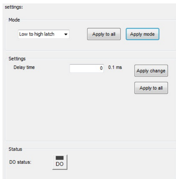
图 2-41 WTD678C 输出上升锁定模式主界面
