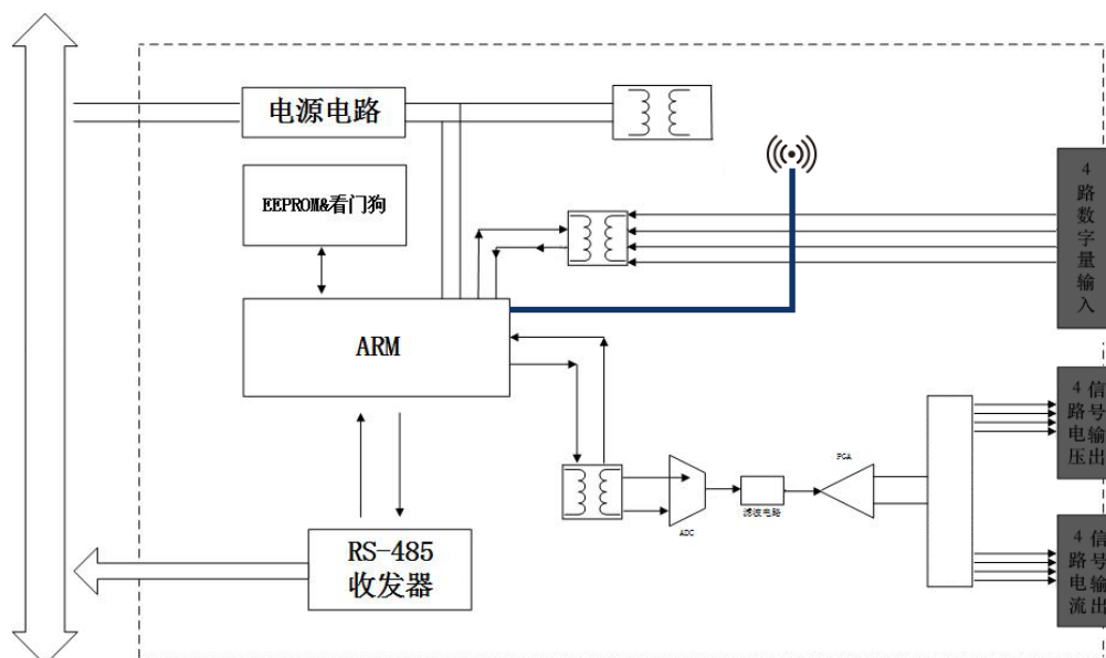
图 3-16 WTD624X 原理框图
