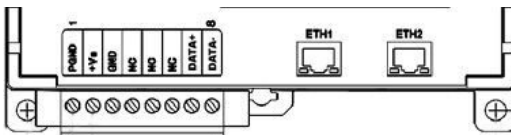
图 3-49 WTD634G 网关接线方式
