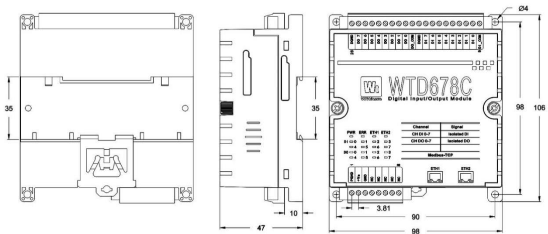
图 1-5 WTD4XXX 模块安装尺寸图
