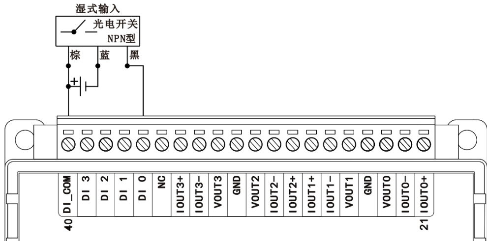
图 3-21 WTD624X NPN 型湿式输入接线方式
