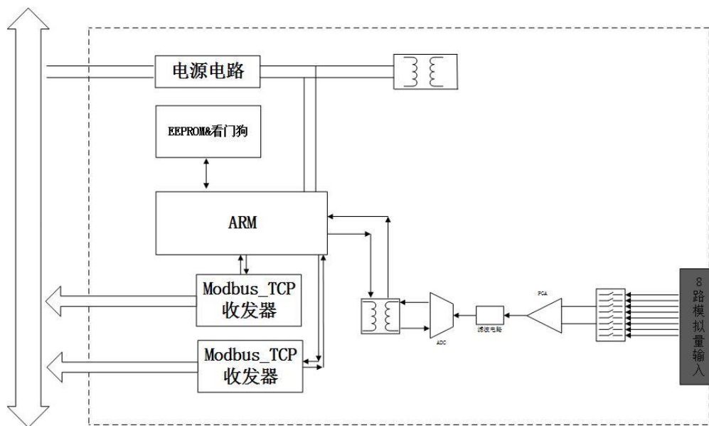
图 3-9 WTD618X 原理框图
