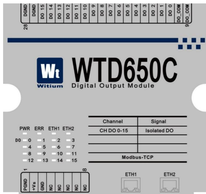
图 3-32 WTD650C 端子功能排列
