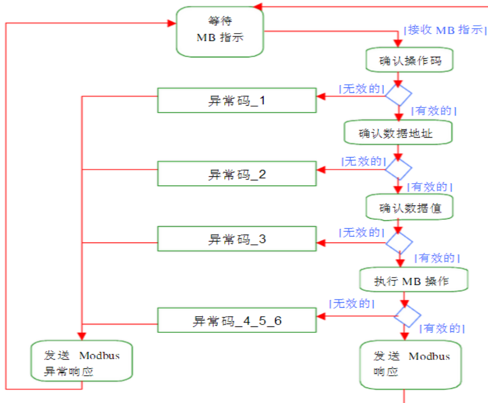
图 4-4 MODBUS 事务处理的状态图
