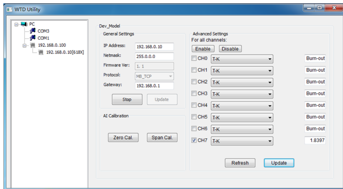
图 2-11 WTD618X 主界面
