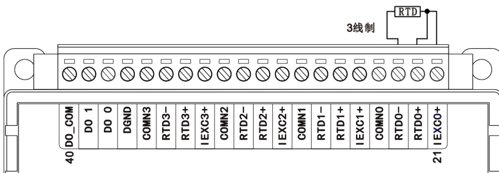
图 3-5 WTD614P 3 线 RTD 接线方式
