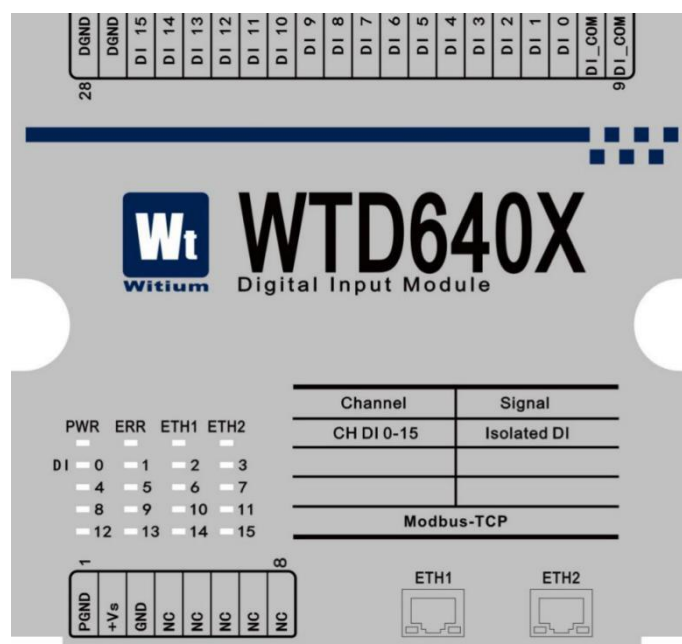
图 3-25 WTD640X 端子功能排列
