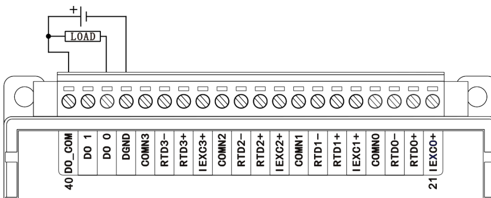
图 3-7 WTD614P 数字量输出接线方式
