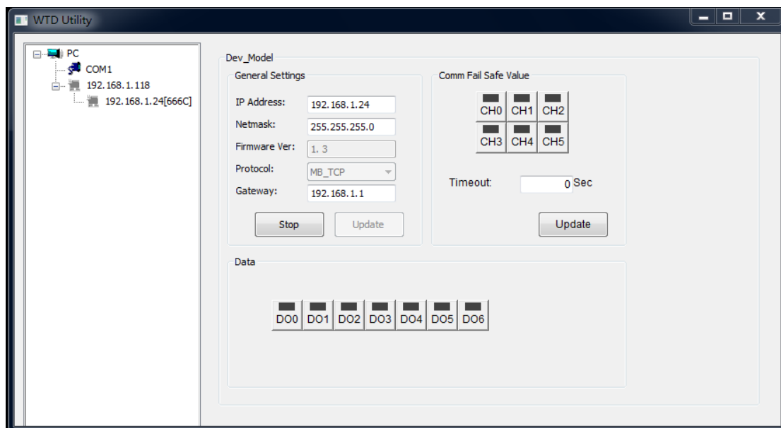
图 2-26 WTD666C 主界面
