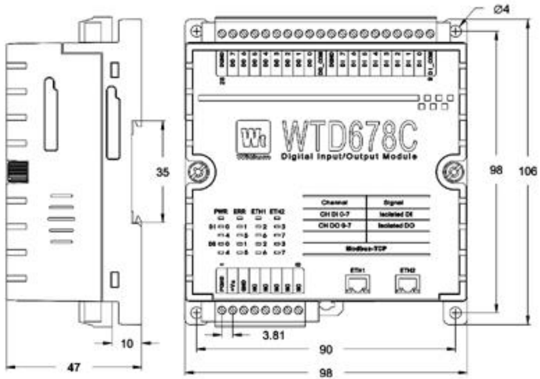
图 1-4 WTD6XXX 模块安装尺寸图
