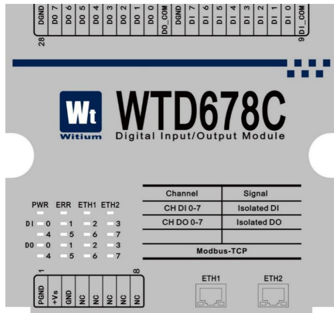
图 3-40 WTD678C 端子功能排列
