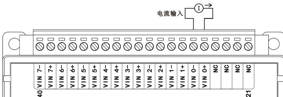
图 3-12 WTD618X 电流输入接线方式 1
